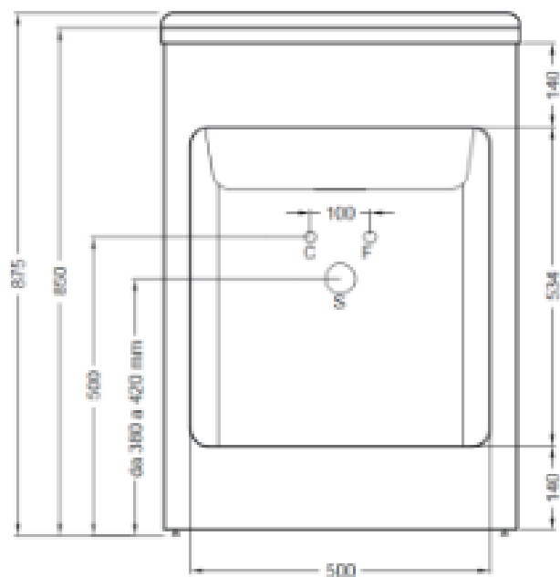
VISTA FRONTALE
