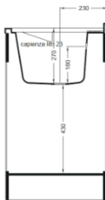
SEZIONE A-A
